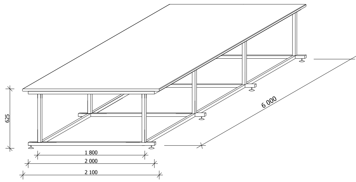
Стол раскроечный
